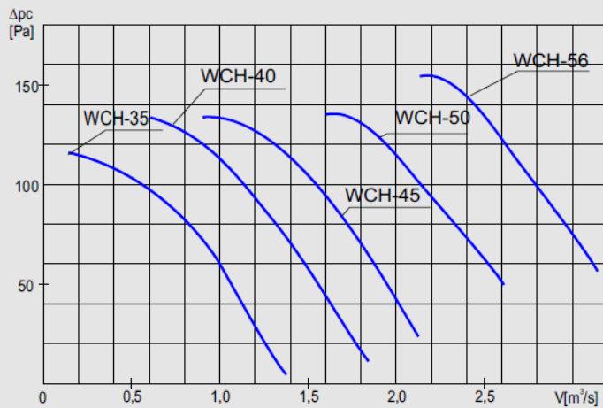
Charakterystyka aerodynamiczna WCH
