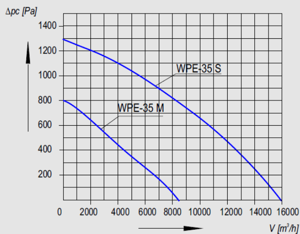
Charakterystyka aerodynamiczna WPE-35
