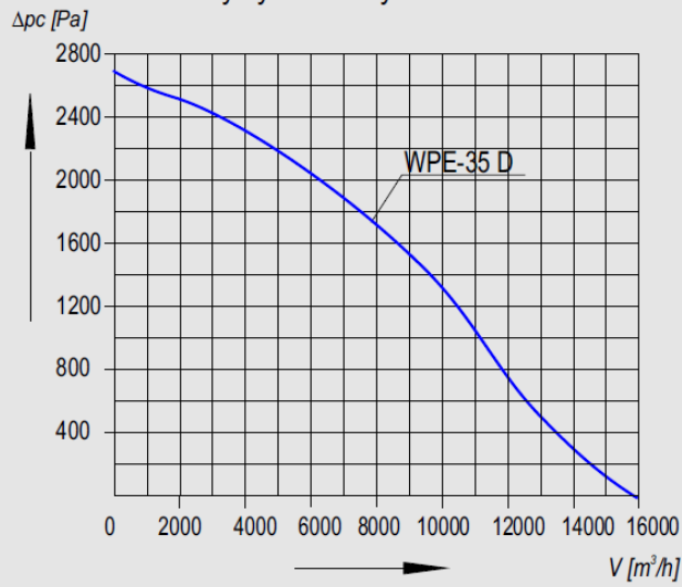
Charakterystyka aerodynamiczna WPE-35 D
