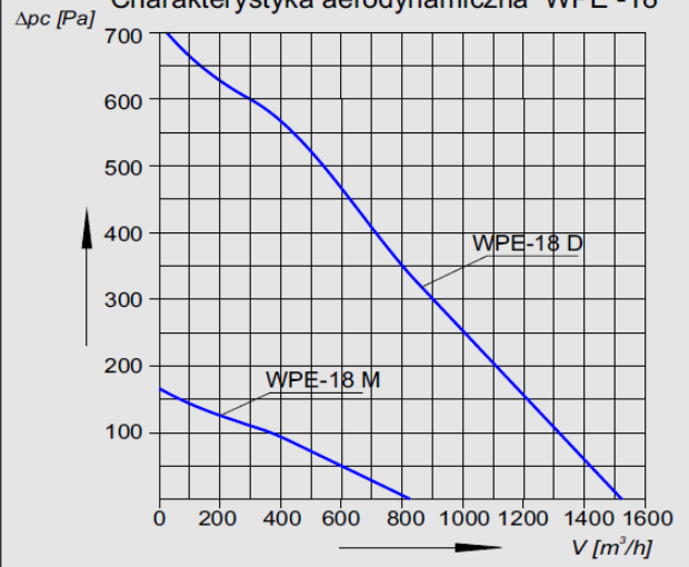
Charakterystyka aerodynamiczna WPE -18
