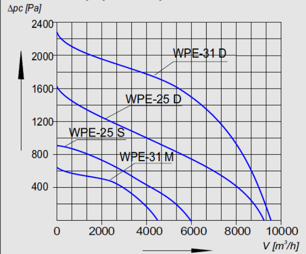
Charakterystyka aerodynamiczna WPE-25,31
