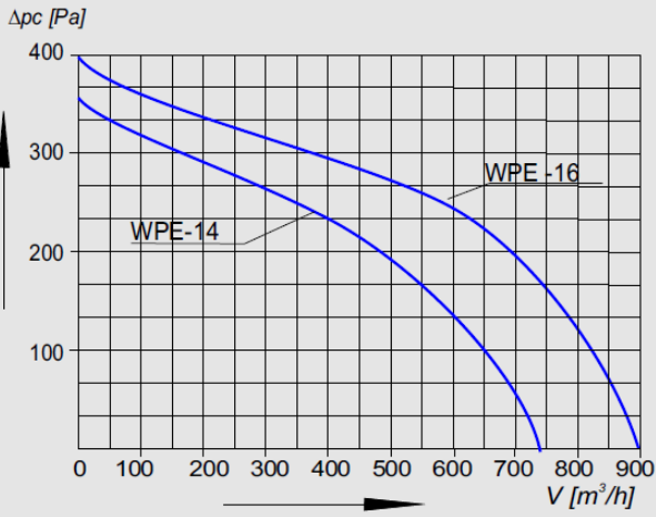
Charakterystyka aerodynamiczna "WPE-14,16"
