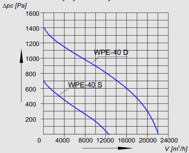
Charakterystyka aerodynamiczna "WPE-40"
