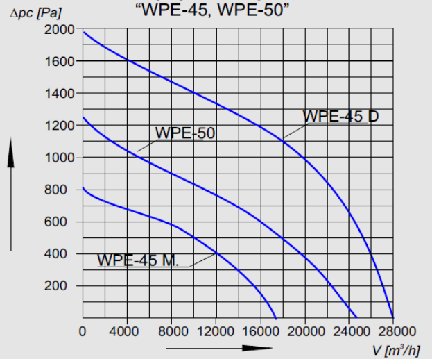
Charakterystyka aerodynamiczna "WPE-45, WPE-50"
