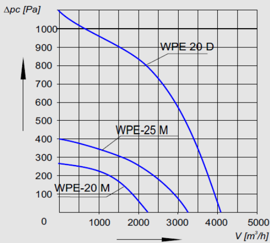
Charakterystyka aerodynamiczna WPE-20
