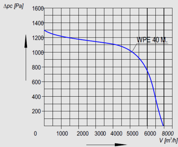
Charakterystyka aerodynamiczna WPE- 40 M
