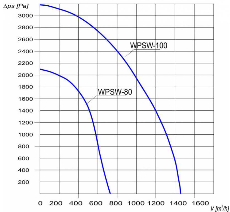
Charakterystyka aerodynamiczna WPSW-80, WPSW-100
